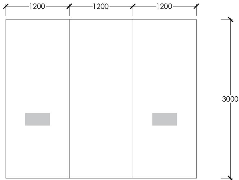
Figura 2_Prospecto controparete con scatole elettriche - vista lato camera ricevente
