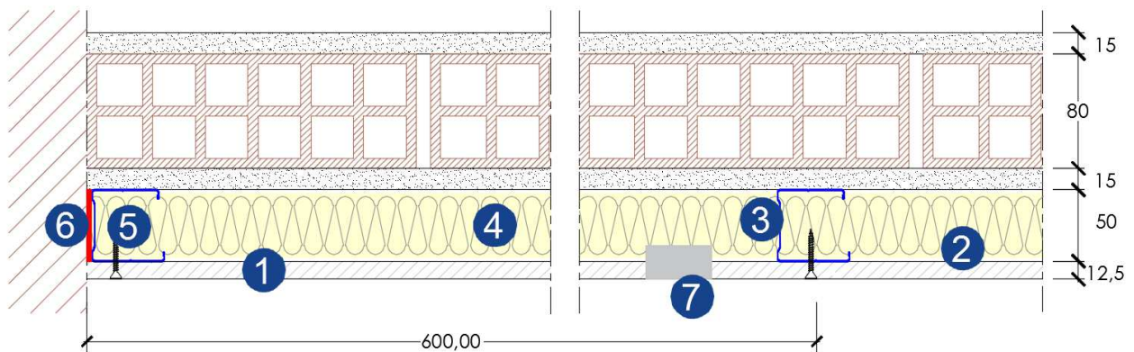
Figura 3_Disegno tecnico del campione: sezione - estremità (*)
