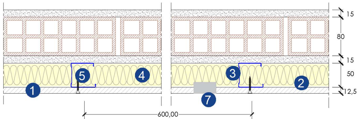
Figura 4_ Disegno tecnico del campione: sezione - parte centrale (*)
