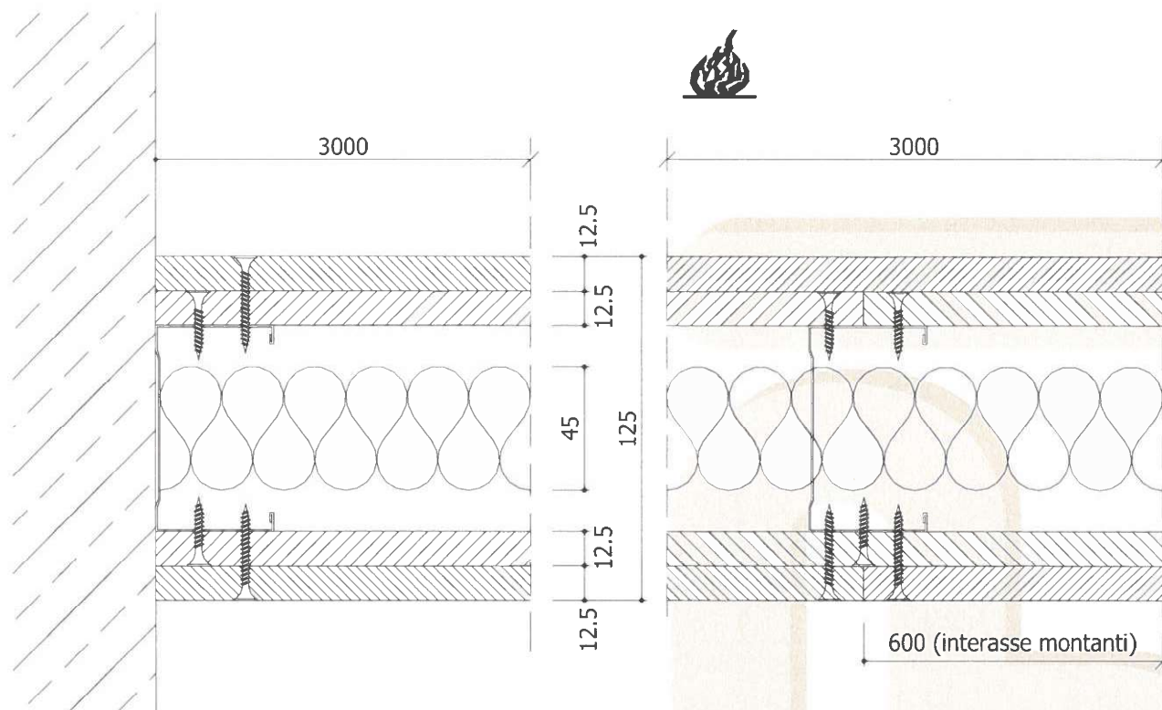
Sezione orizzontale del campione in prova
