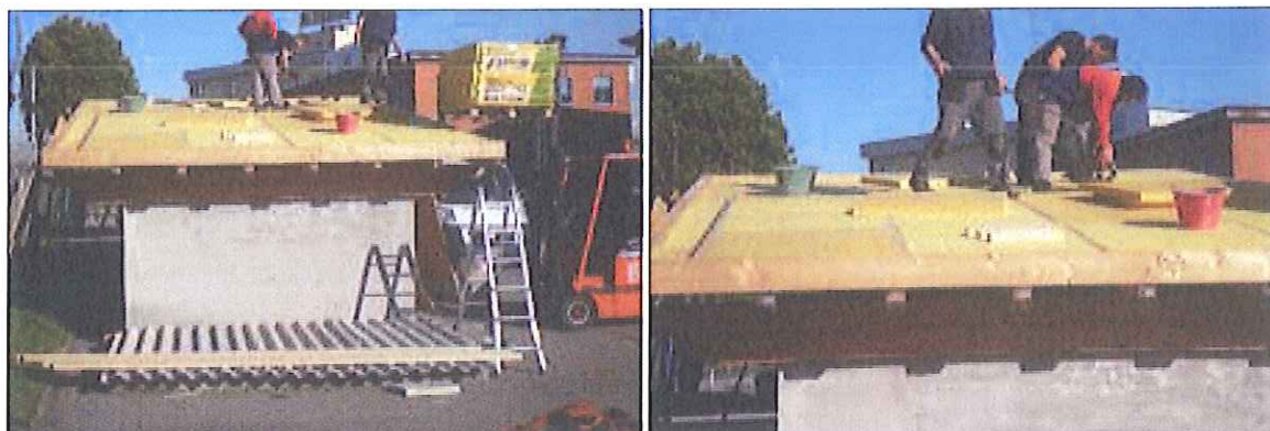
Figura 8 – Particolari di posa della configurazione provata: SUPERBAC N Roofline® con doppia orditura incrociata
